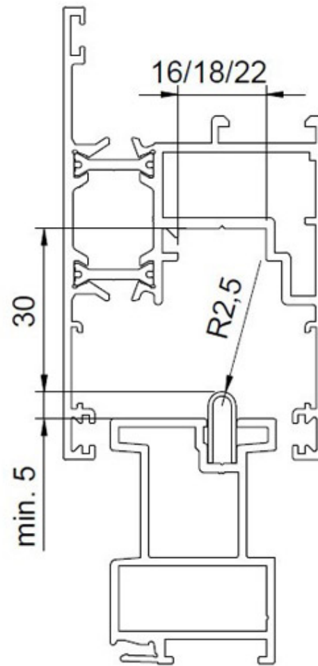
Modèle 400 kg
